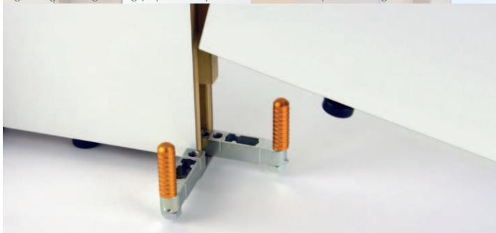
Wandmodul Leichtbau mit Verbinder und Stellfüßen Lightweight wall panel with connectors and adjustable feet
