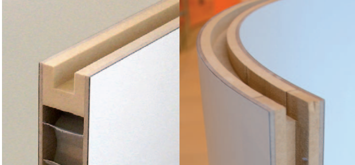
Leichtbau mit Papierwabe lightweight design using paper honeycomb
