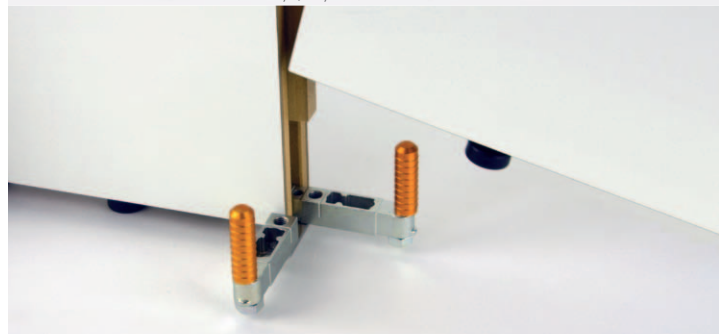
Fixierung des G40 Verbinders mit Federtechnik G40 connector fixed with tounge technology
